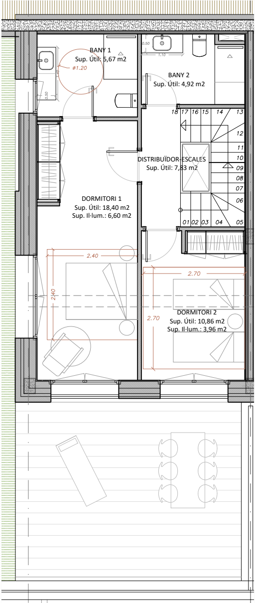
PLANTA PRIMERA
