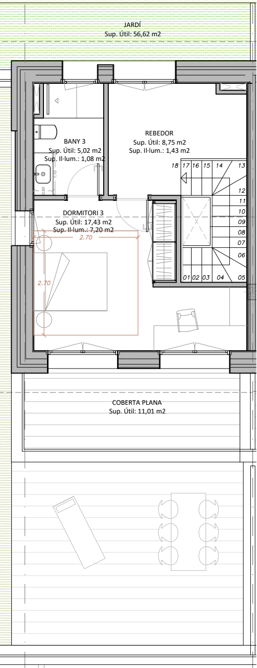
PLANTA SOTACOBERTA
